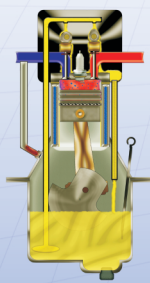
Cirkulace oleje po výměně oleje s provedením vnitřním čištěním motoru
